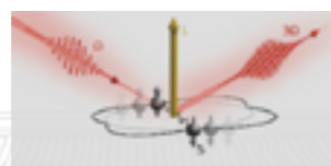
铜基高温超导中的希格斯波色子 (Higgs boson)
