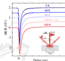
时间分辨/超快光谱学
