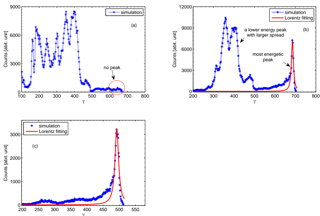
图2-4 电子束能谱，对应于 (a) 单级 L_1 = 200 \mu\text{m} ，(b) 两级， L_1 = 135 \mu\text{m} ， L_2 = 1000 \mu\text{m} ，(c) 两级， L_1 = 135 \mu\text{m} ， L_2 = 400 \mu\text{m} 。(a) 中 \gamma = 600 \sim 700 段没有峰，因为气体密度包络没有进行优化。(b) 中有能量 350 MeV，能散度为 1.62% 的单能峰，同时包含一个较低能量，较大能散的准单能峰。为了去除这个能量较低的峰，我们将 L_2 调至 400 \mu\text{m} ，于是得到了 (c) 中的单峰能谱。
