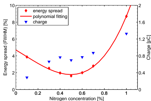
图 2-7 最高能峰的能散度 (菱形) 和电荷量 (三角形) 与氮气浓度 c\% 的关系。其他参数为 L_1 = 135 \mu\text{m} , L_2 = 1000 \mu\text{m} , L_3 = 100 \mu\text{m} 。
