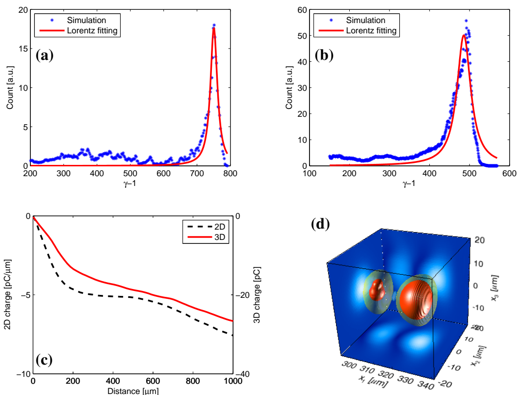
图 3-6 参数优化后的二维平板几何模拟，以及三维模拟。(a) 二维模拟所得输出电子束能谱，使用优化后的激光参数 a_0 = 2.9 , k_p W_0 = 5.228 。(b) 三维模拟所得输出电子束能谱，使用的参数为，氦气密度 n_{\text{He}} = 8 \times 10^{-4} n_c ，归一化激光矢势 a_0 = 2.3 ，归一化腰斑半径 k_p W_0 = 4.066 。能谱在加速距离为 1.56 mm 处测量。(c) 上述二维和三维模拟中注入电子束的电量随激光传播距离的变化。(d) 三维模拟中尾场伪势 \psi 的等值面图，以及它向各个侧面的投影图。三维模拟中整个模拟盒尺寸与二维模拟相同，但是图中只显示了中心区域。
