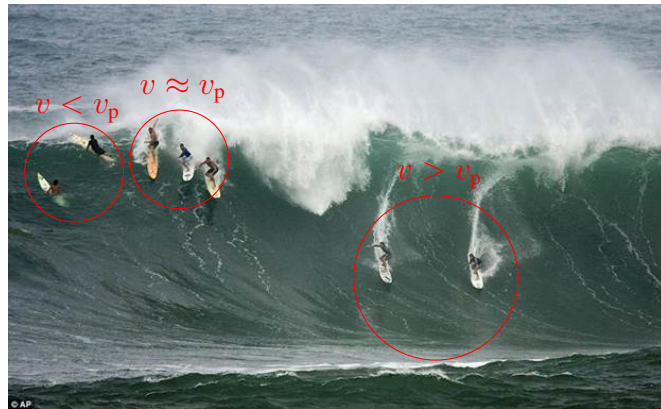
图 1-5 冲浪与捕获示意图。假设一段时间内浪具有恒定的相速度 v_p 。图中最左边两个人在接近浪的顶点（势能极大值点）时的速度仍小于 v_p ，他们将从加速相位跨过顶点进入减速相位而无法获得持续加速，即未能被浪捕获。中间三个人在接近浪的顶点具有的速度接近或者略大于 v_p ，他们能持续处在加速相位很长一段时间而获得持续加速，即已经被浪捕获。最右边两个人速度已经大于 v_p ，他们在持续从浪获得动能的同时速度越来越快，因此在浪的参考系下向前移动；当他们到达浪的底部时就无法再获得更多的动能，称为失相。图片来自网络。
