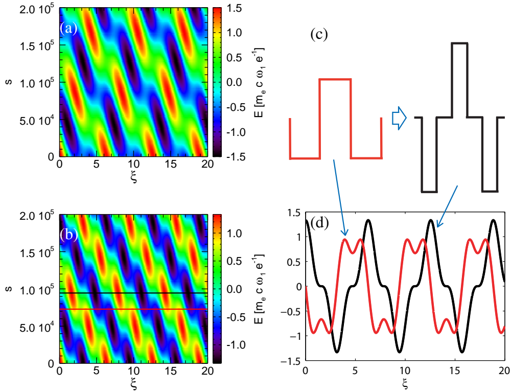
图 4-2 根据式 (4-3) 作出的等离子体中传播的双色激光电场演化图。(a) 参数为 a_{10} = 1 , a_{20} = 1/4 , \omega_2/\omega_1 = 2 , \omega_p/\omega_1 = 0.01 。(b) 参数为 a_{10} = 1 , a_{20} = 1/9 , \omega_2/\omega_1 = 3 , \omega_p/\omega_1 = 0.01 。(c) 使用 SWBL 组合原因的示意图。(d) 在 (b) 中选取的两个截线 (黑线和红线) 上电场值的振荡曲线。这两条截线都是选取 s 为定值。
