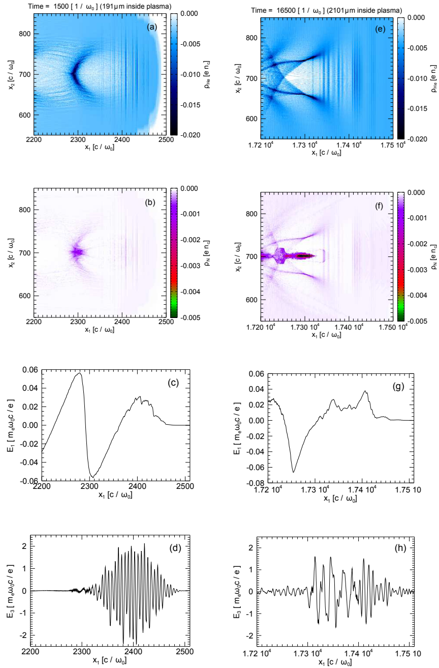
图 2-3 两个不同时刻的激光尾波场和空泡结构。图 (a) 到 (d) 是在模拟时间为 1500 处 (传播距离 191 \mu\text{m} )，图 (e) 到 (h) 是在模拟时间为 16500 处 (传播距离 2101 \mu\text{m} )。 (a) 和 (e) 是从氦气和氮气中电离的电子密度图，其中没有注入，而 (b) 和 (f) 是从氮气中电离的电子密度图，其中有注入。注入电子来自氮气原子的 K 层电子电离。(c) 和 (g) 展示了纵向电场，(d) 和 (h) 展示了沿轴的激光场。
