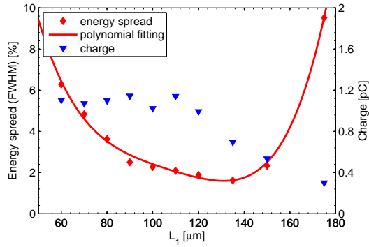
图 2-5 最高能峰的能散度 (菱形) 和电荷量 (三角形) 与 L_1 的关系。其他参数为 L_2 = 1000 \mu\text{m} , L_3 = 100 \mu\text{m} , c\% = 0.5\% 。
