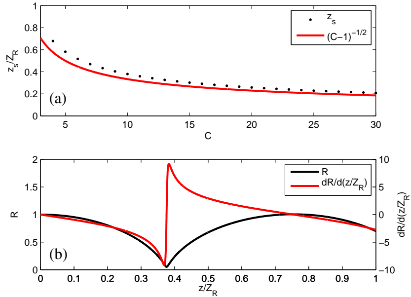
图 3-1 二维平板几何下激光包络半径演化曲线。(a) 半演化周期长度 z_s 随参数 C 的变化，以及其与柱对称几何情况下的对应解析值 (C - 1)^{-1/2} 的对比。(b) 一个典型的 C 取值时的 R 和 \dot{R} 演化曲线。
