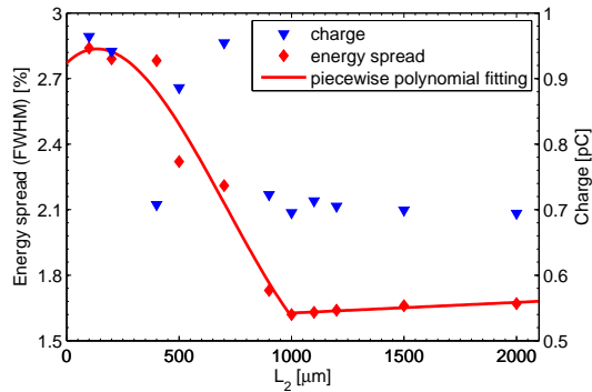
图 2-6 最高能峰的能散度 (菱形) 和电荷量 (三角形) 与 L_2 的关系。其他参数为 L_1 = 135 \mu\text{m} , L_3 = 100 \mu\text{m} , c\% = 0.5\% 。
