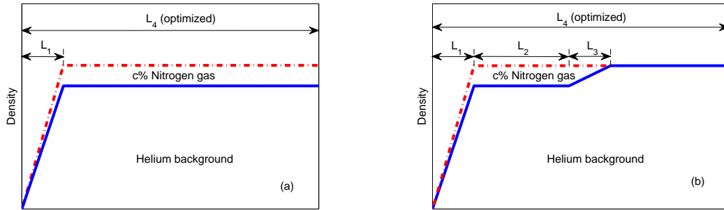
图 2-2 单级 (a) 以及两级 (b) 加速模拟的电子密度示意图。粗线表示电子密度包络。激光从左侧入射。(a) 气体靶为氦-氮混合气体，密度上坡长度为 L_1 ，氮气浓度 c\% 。(b) 第一级密度上坡长度 L_1 ，平台区域长度 L_2 。两级之间密度转换区域长度 L_3 。优化 L_4 使得粒子束能散演化到最小。第一段氮气浓度 c\% 。两段电子总密度相等。
